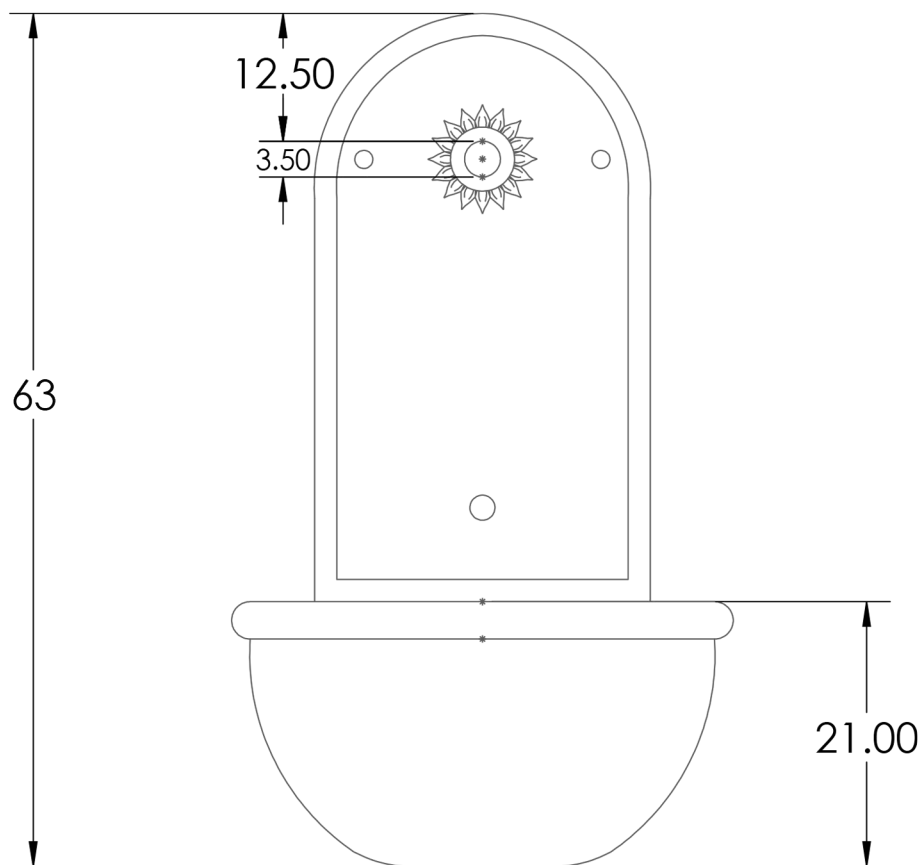
Elülső nézet
